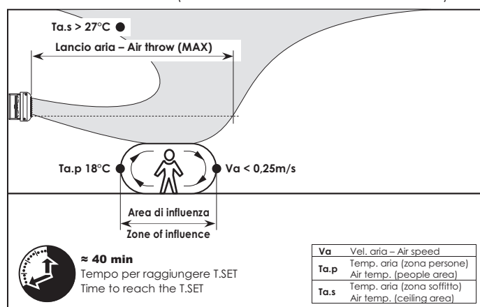
Aerotermostando standard (SENZA DIFFUSORE di mandata "Venturi-Jet-Induction") Standard Aerotherm (WITHOUT DIFFUSER "Venturi-Jet-Induction")
