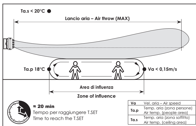
Aerotermostando CON DIFFUSORE di mandata "Venturi-Jet-Induction" Aerotherm WITH DIFFUSER "Venturi-Jet-Induction"
